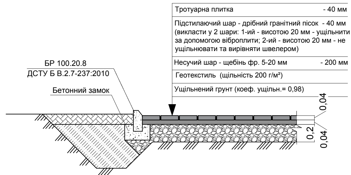
Пішохідна доріжка з покриттям із плитки ФЕМ (тип Б)
